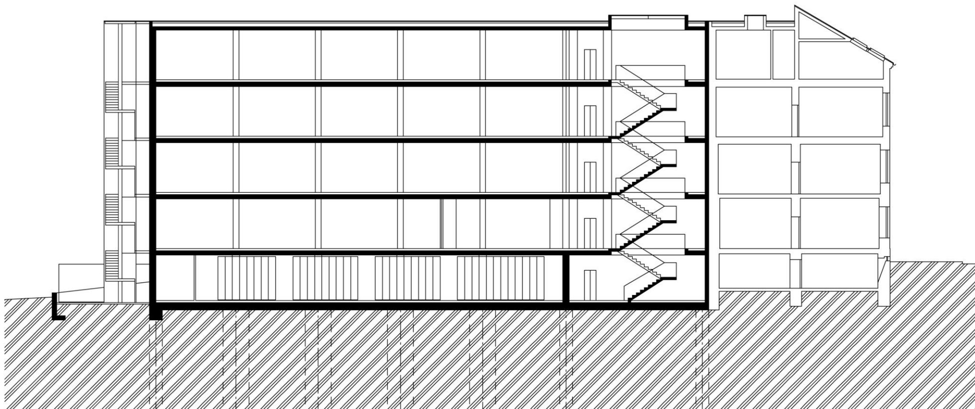
PODÉLNÝ ŘEZ
