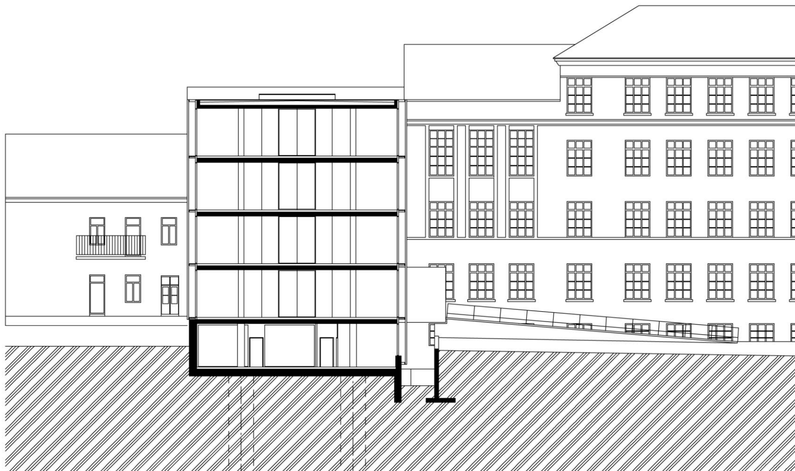
PŘÍČNÝ ŘEZ
